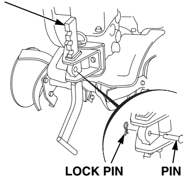
DRAG BAR
