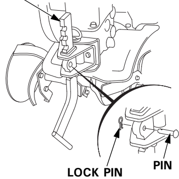
DRAG BAR
